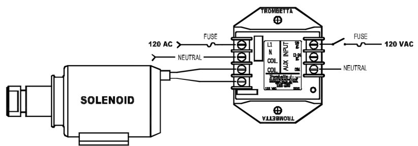
S500-A300 MODULE
